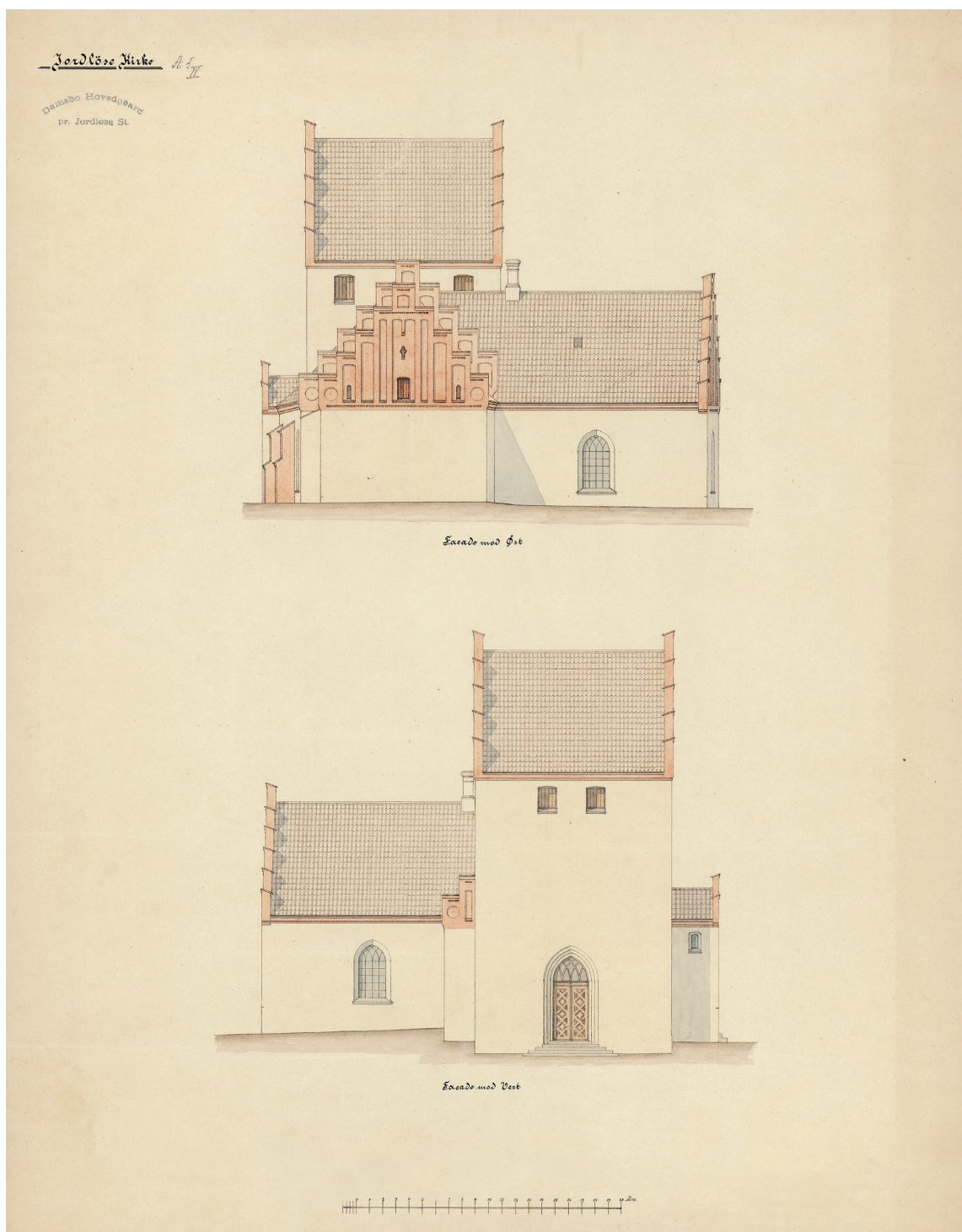
Fig. 14g-h. Forslag til restaurering o. 1899. 1:300. g. Østfacader. h. Vestfacader. I NM. – Proposal for restoration, c. 1899. g. East facades. h. West facades.
