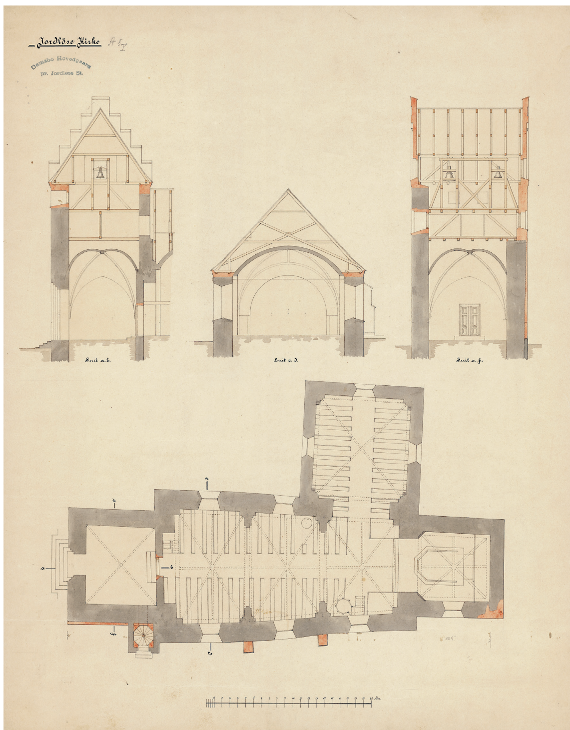
Fig. 14a-d. Forslag til restaurering o. 1899. 1:300. a. Tværsnit af tårn set mod nord. b. Tværsnit af tårn set mod øst. c. Tværsnit af vestforlængelse set mod øst. d. Grundplan. I NM. — Proposal for restoration, c. 1899. a. Cross-section of the tower looking north. b. Cross-section of the tower looking east. c. Cross-section of the western extension looking east. d. Ground plan.
