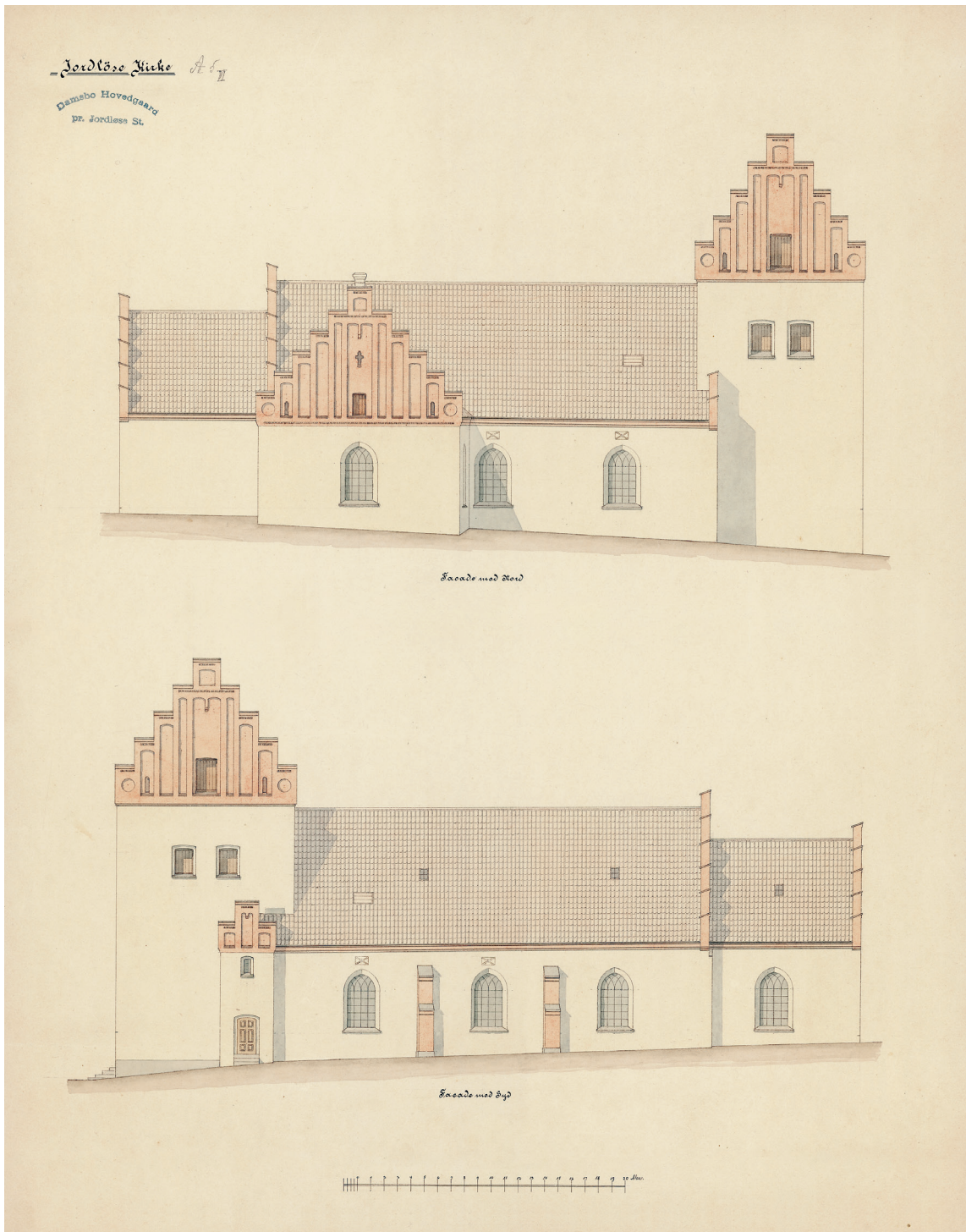
Fig. 14e-f. Forslag til restaurering o. 1899. 1:300. e. Nordfacader. f. Sydfacader. I NM. — Proposal for restoration, c. 1899. e. North facades. f. South facades.
