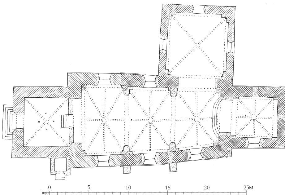
Fig. 7. Grundplan. 1:300. Målt af Lars Mindedal 1969, suppleret og tegnet af Pia K. Lindholt 2025. Signaturforklaring s. 9. – Plan. Key on p. 17.
