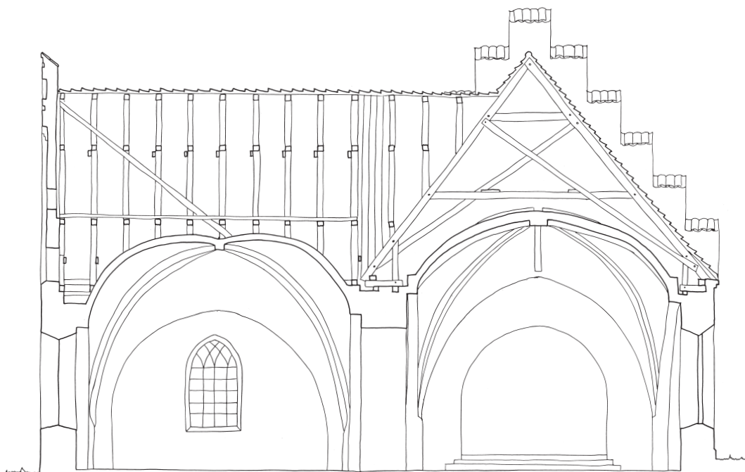
Fig. 6. Tværnsnit. 1:150. Målt og tegnet af Pia K. Lindholt 2025. – Cross-section.
