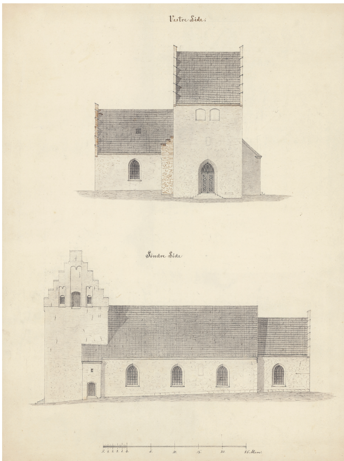
Fig. 12f-g. Opmåling af kirken o. 1880. 1:300. f. Vestfacader. g. Sydfacader. I NM. — Scale drawings of the church from c. 1880. f. West facades. g. South facades.
